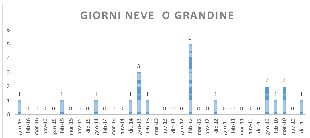
Figura 13 – Giorni di neve o grandine (2010-2016)
